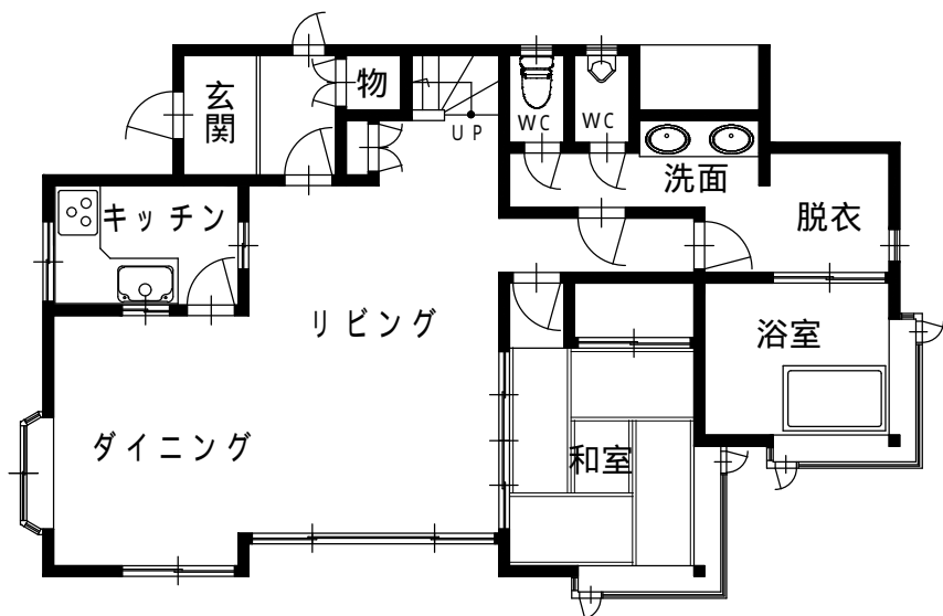
1階平面図
