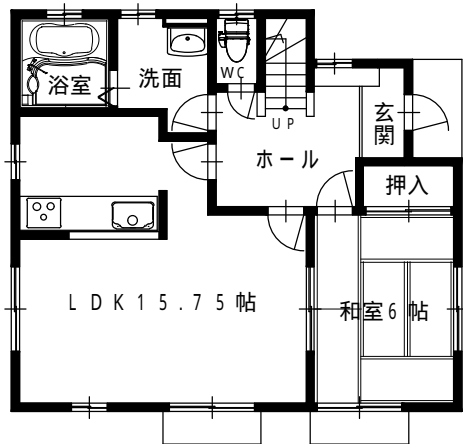
1階平面図
