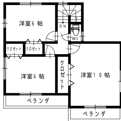
2階平面図
