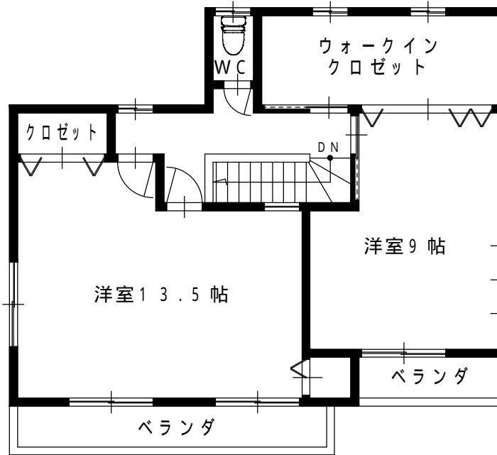
2 階平面図
