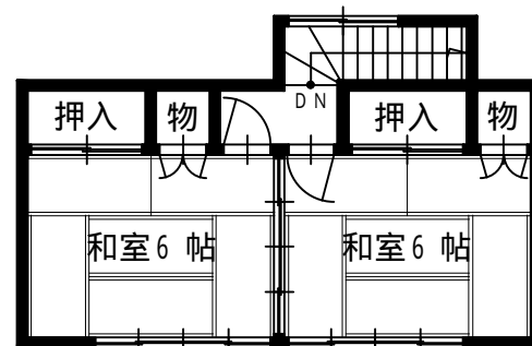
2階平面図
