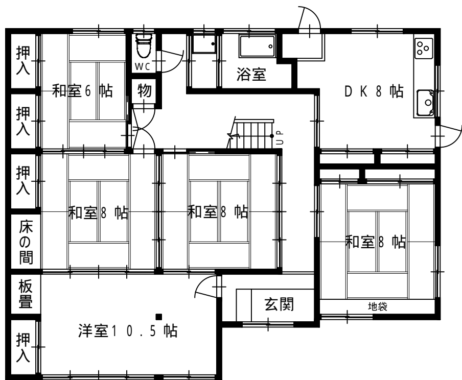
1階平面図
