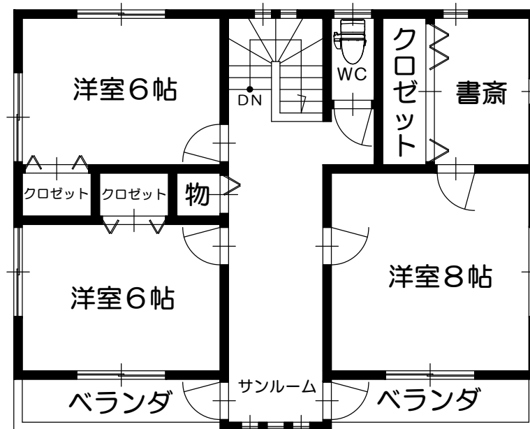
2階平面図
