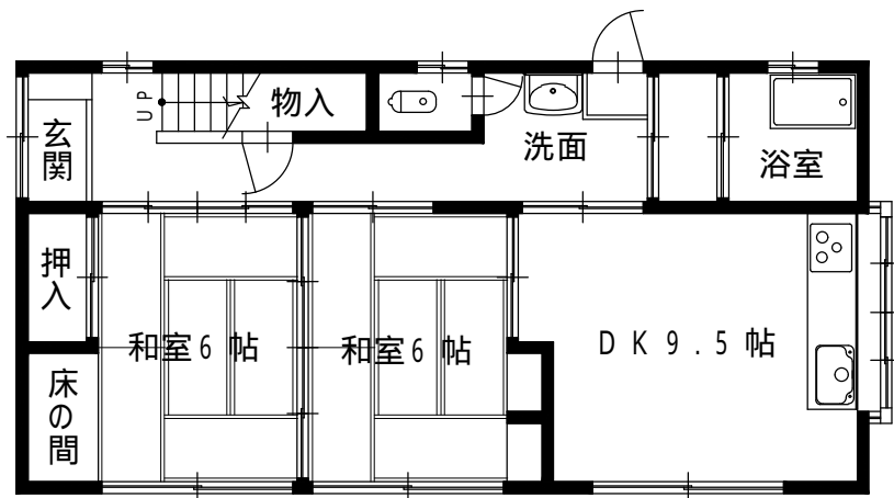
1 階平面図
