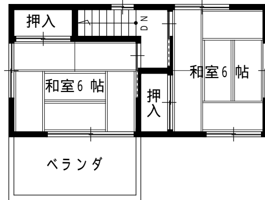
2 階平面図
