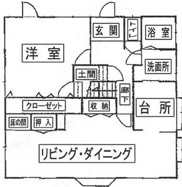
1階平面図
