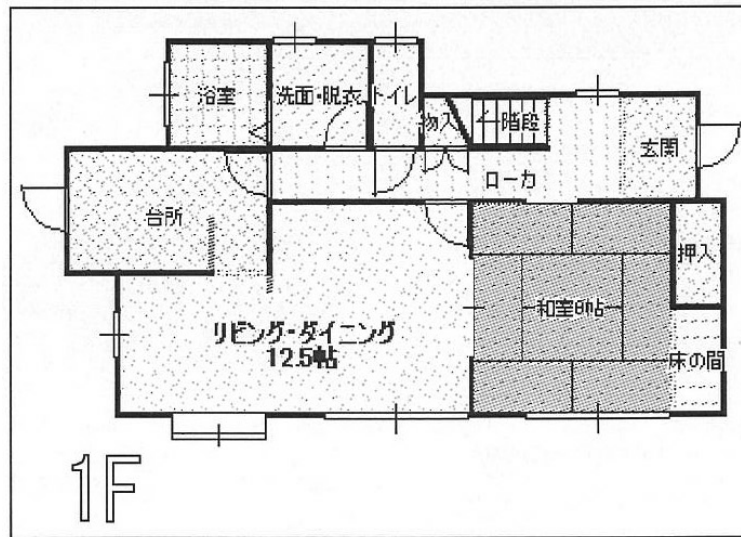
1 階平面図
