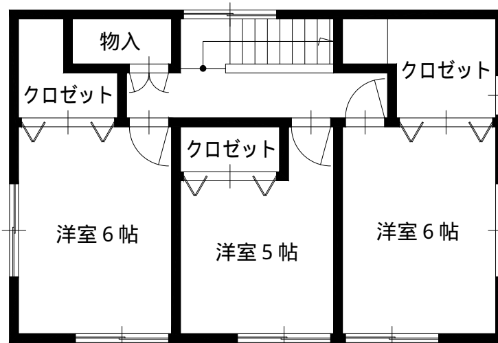
2階平面図
