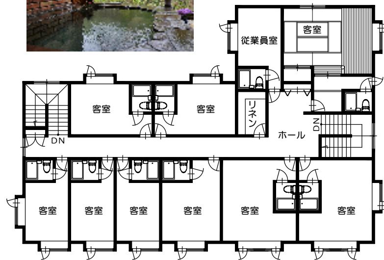
2階平面図
