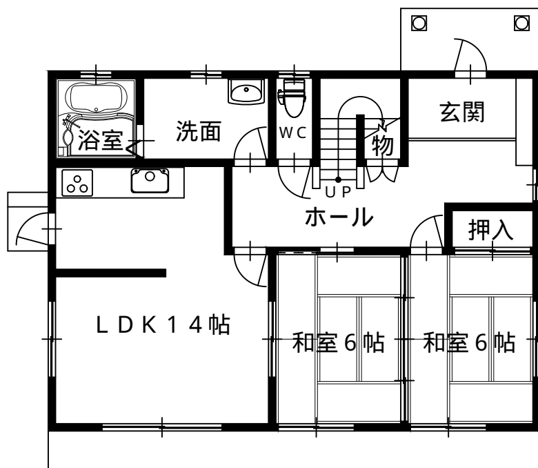
1階平面図
