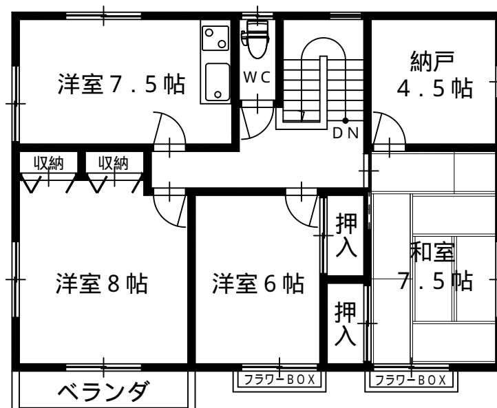
2階平面図
