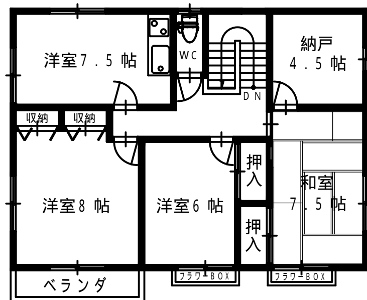
2階平面図
