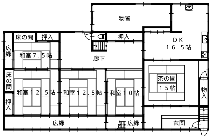
1階平面図
