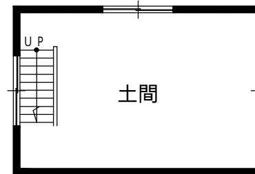
倉庫1階平面図
