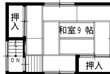
倉庫2階平面図
