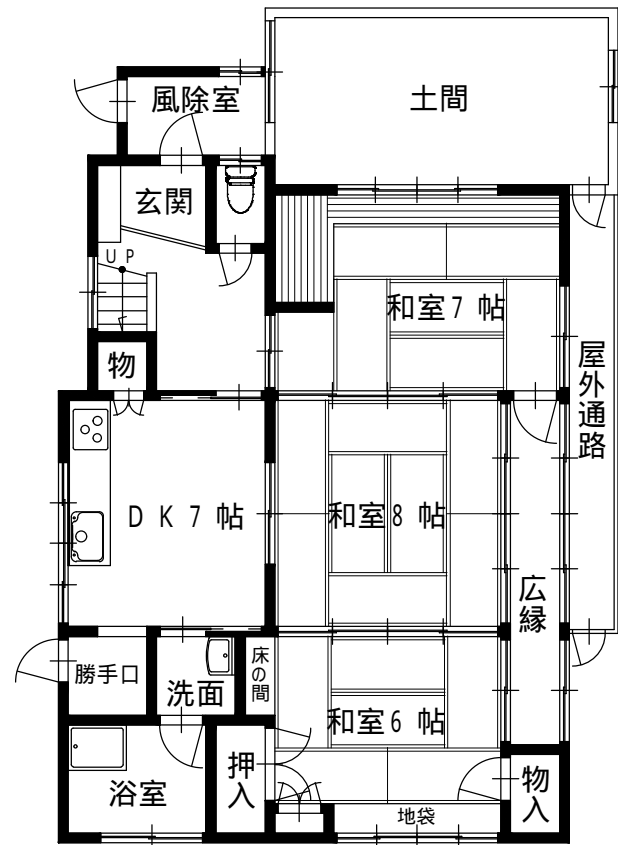
1階平面図
