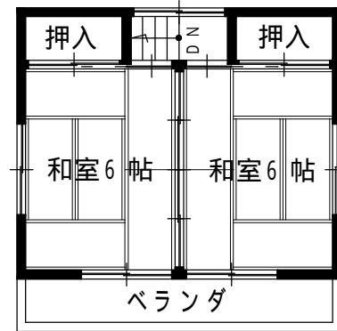
2階平面図
